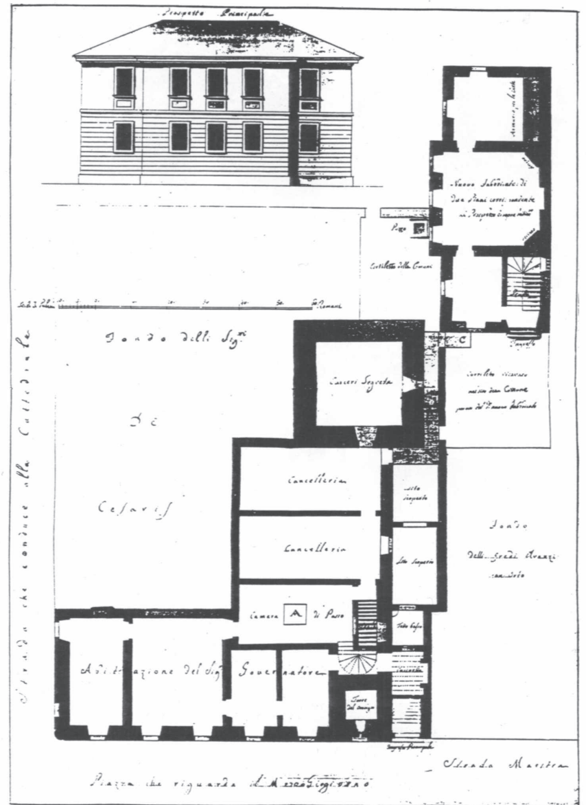
10. L. Campovecchi, Progetto per il restauro del Palazzo Consolare: planimetria , 1828, (ASR, CBG, Serie IV, b. 279, visita dell'avv. Zamboni, 1803, f. 308, appendice n. 64). Cfr. M.T. Valeri, cit. , fig. 7.
