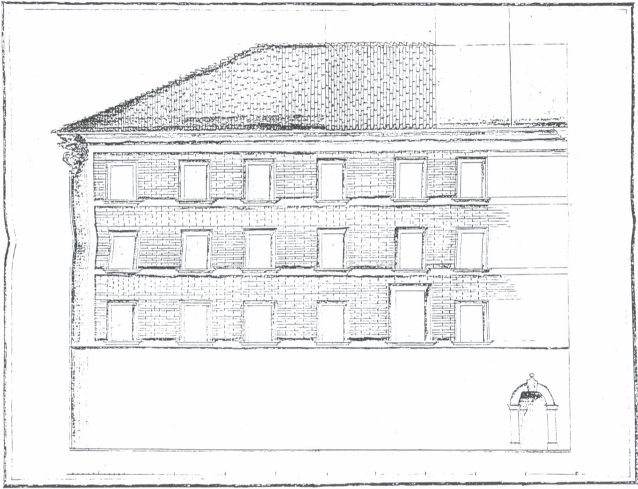
8. Pietro Cocumelli, Progetto per il restauro del Palazzo Consolare di Ferentino: prospetto , 1792, (ASR, CBG, Serie II, b. 1574). Cfr. M.T. Valeri, cit. , fig. 4.
