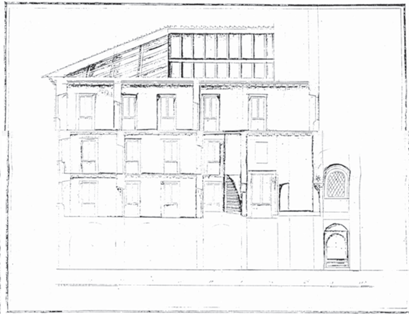
9. P. Cocumelli, Progetto per il restauro del Palazzo Consolare: sezione , 1792, (ASR, CBG, Serie II, b. 1574). Cfr. M.T. Valeri, cit. , fig. 5.
